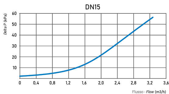
Curve perdita di carico / Pressure loss curves
