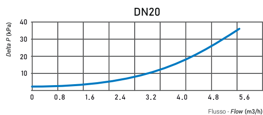
Curve perdita di carico / Pressure loss curves
